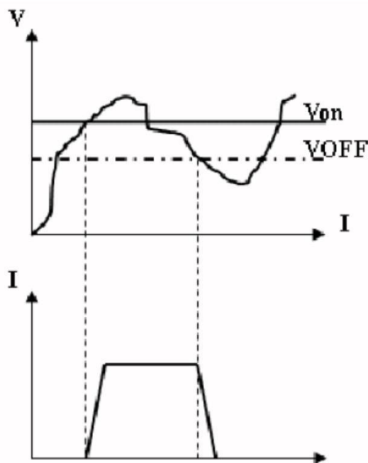
Von / Voff 带载电流波形
